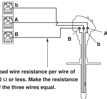
RTD input
