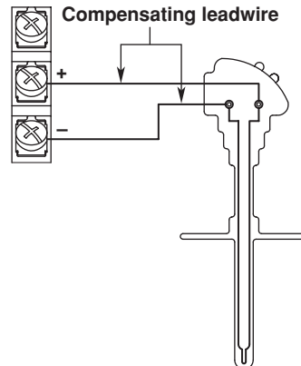
TC input
